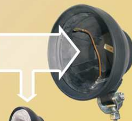
BOITIER GOMME PHARE ROND 63.- HT Art. 98G 127 179-001 • Ø 156 mm
