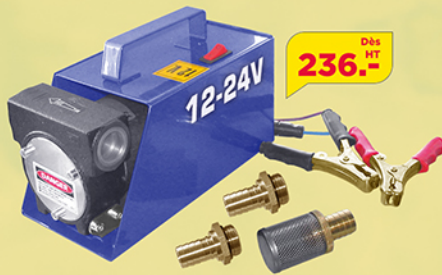
Pompe de transfert 38 l/min • 12 V - 22A Art. 34008 • 24 V - 11A Art. 57541
